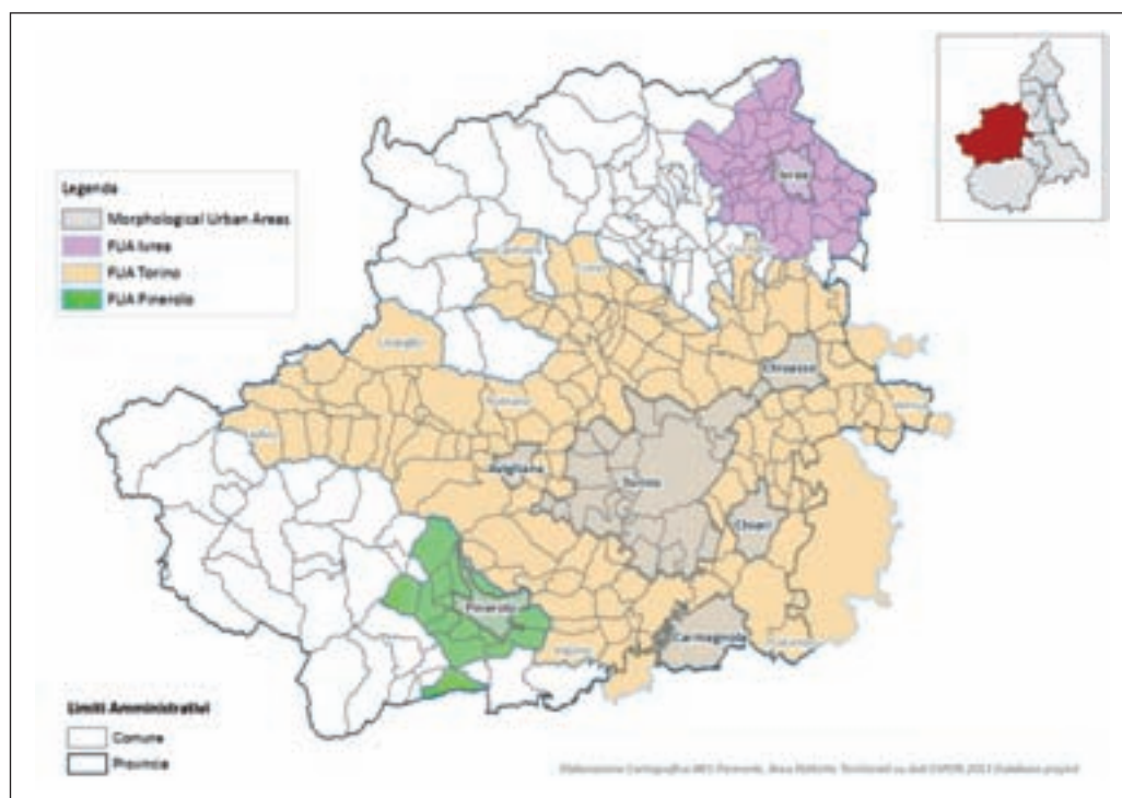
Figura 1 MUA e FUA individuate dall'ESPON in Provincia di Torino (Fonte: Espo Database 2013)
